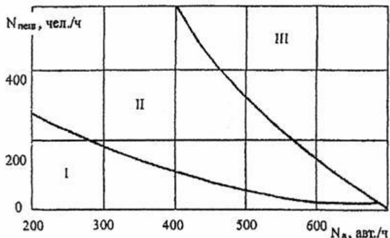
I – нерегулируемые переходы; II – переходы со светофорным регулированием; III – пешеходные переходы в разных уровнях (надземные и подземные) Рисунок 6.1 – Области применения пешеходных переходов различных типов
